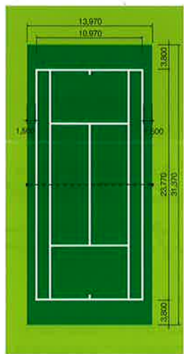
サイド0.9m/バック3.5m張り替え ●面積：約438㎡/面 ●標準施工日数：2～3日/面
