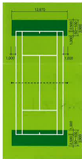
ベースラインまわり張り替え ●面積：約100㎡/面 ●標準施工日数：1～2日/面
