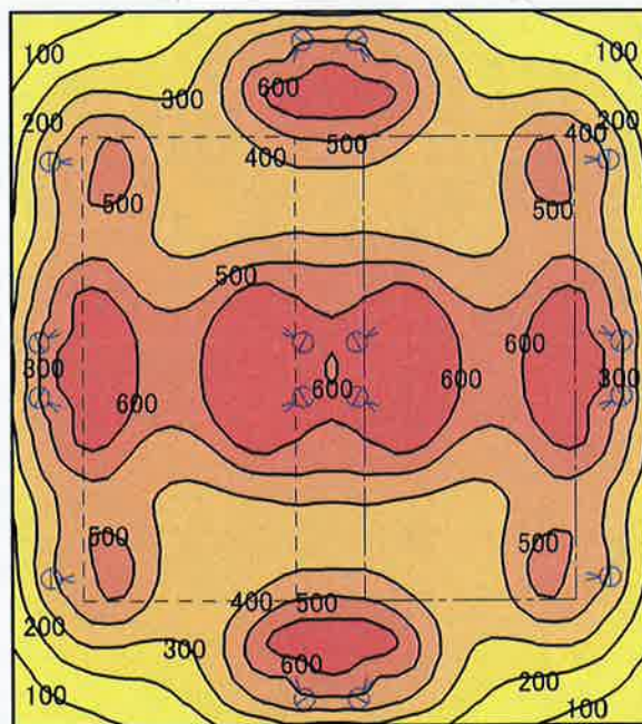
参考照度分布図
